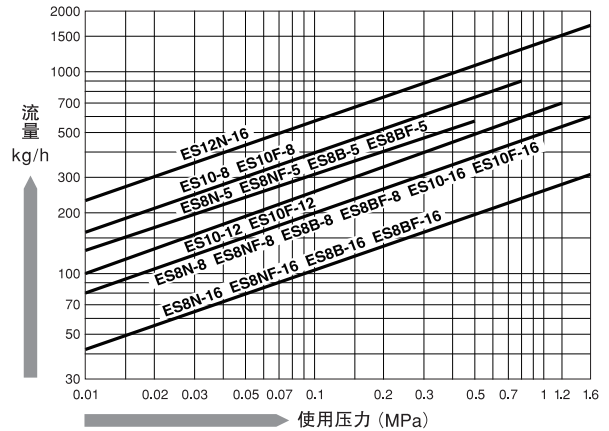
ES8N · ES8B · ES10 · ES12N-流量图
