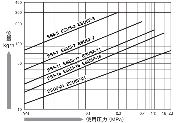
ES5 · ESU5-流量图
